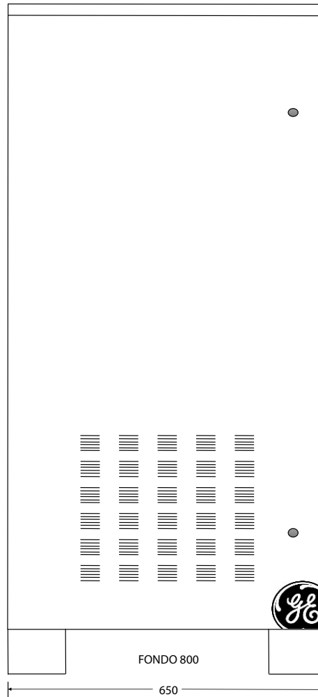
GABINETE DE TRANSFORMADORES
